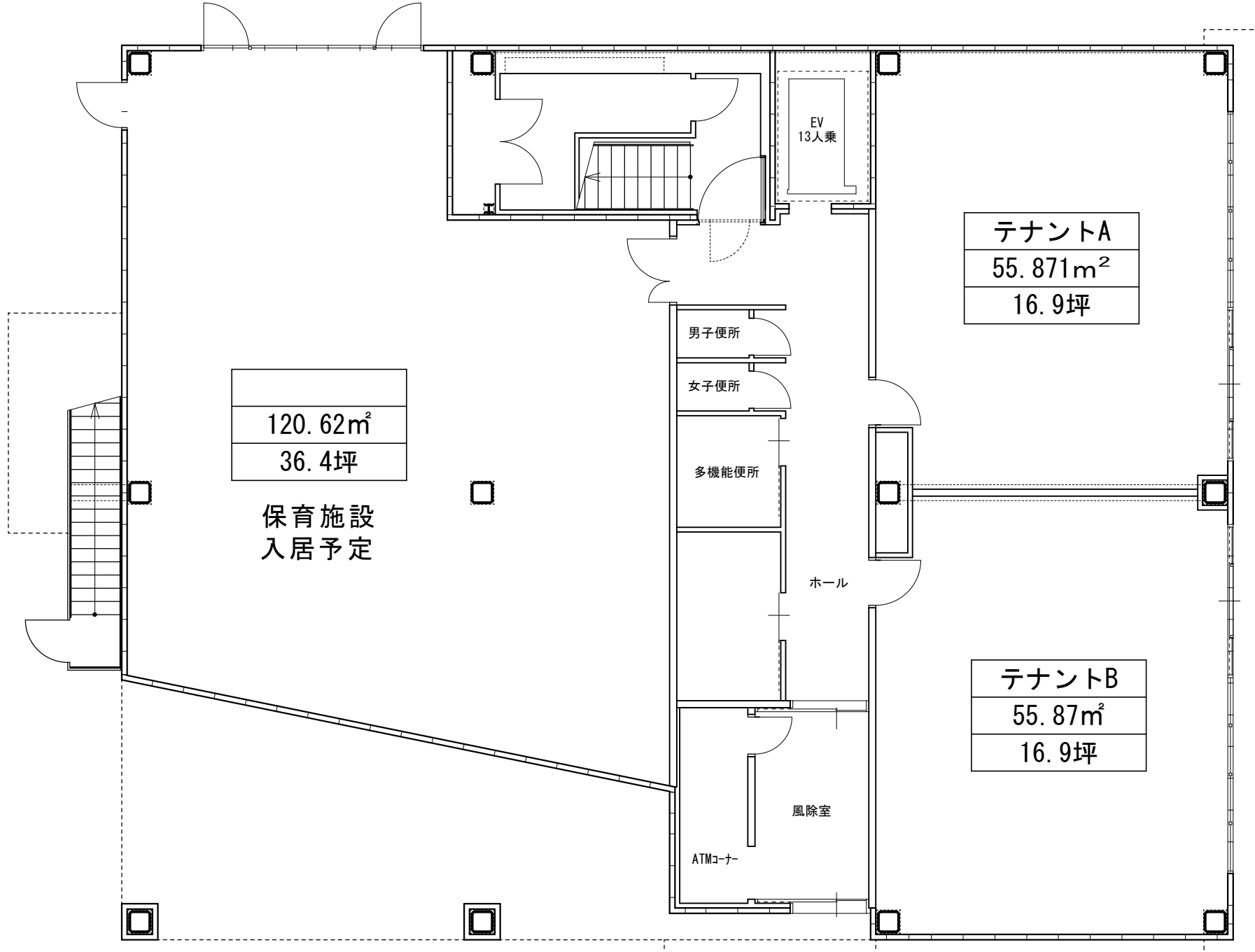
1階 平面図
