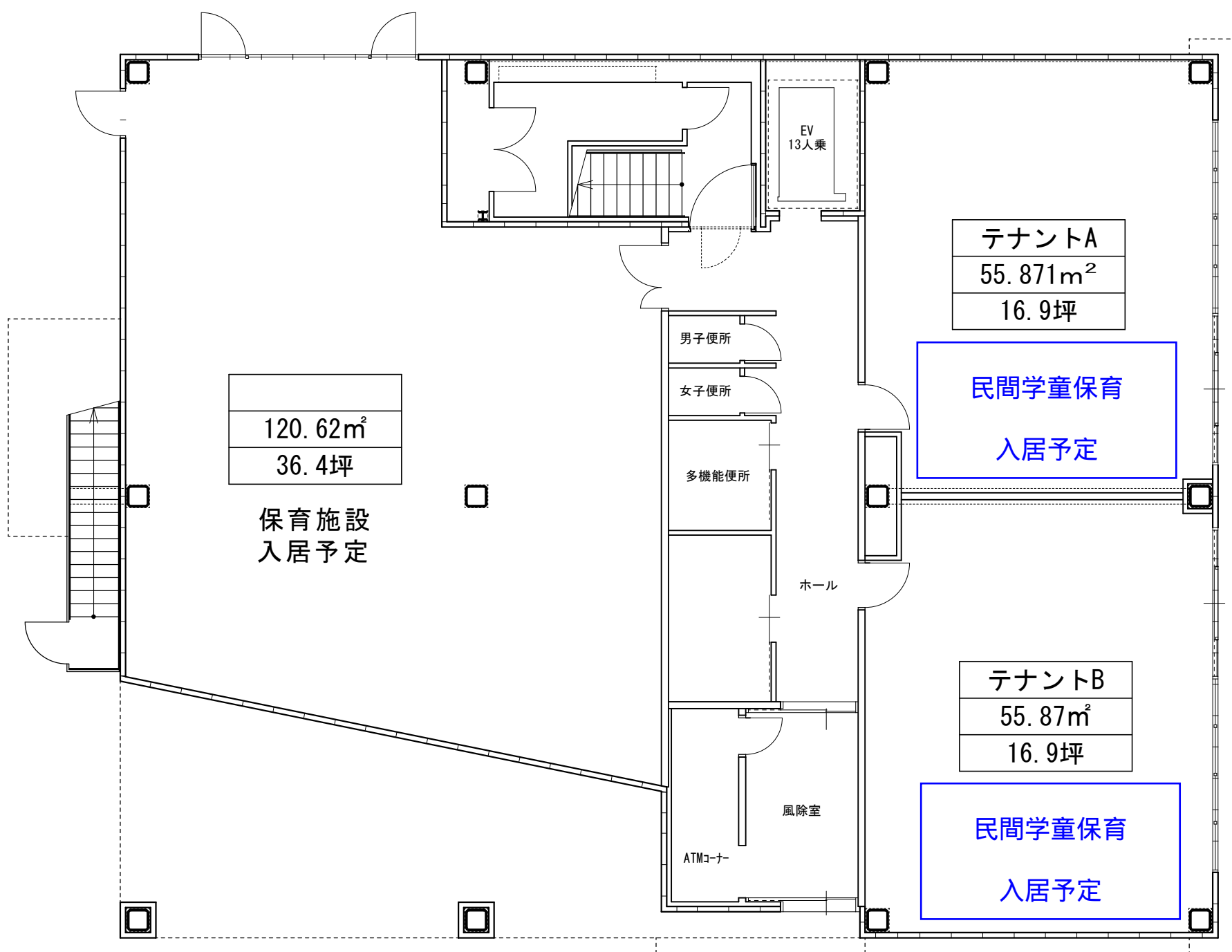
1階 平面図
